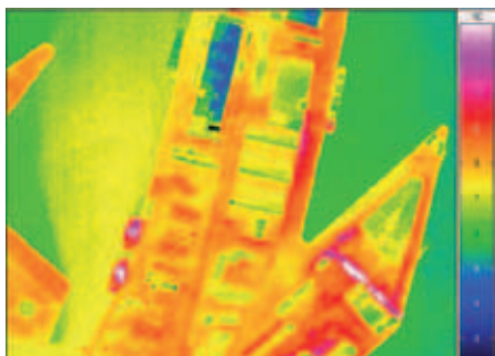
Billedet viser havnen fra Århus. Temperaturforskellen mellem blå og røde farver er ca. 4-6 grader.
